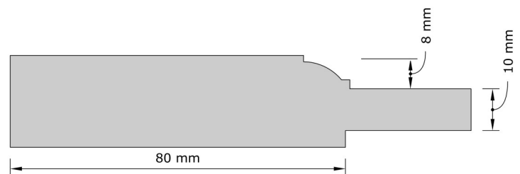
OVOLO
